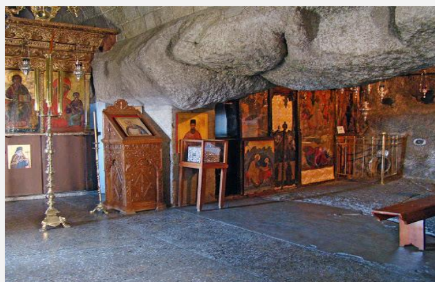
Σπήλαιο Αποκάλυψης
