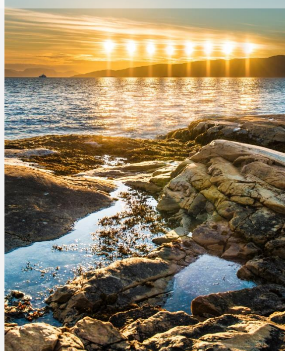
Φάσεις του Ηλίου κατά τη διάρκεια του φαινομένου του Ήλιου του Μεσονυχτίου
